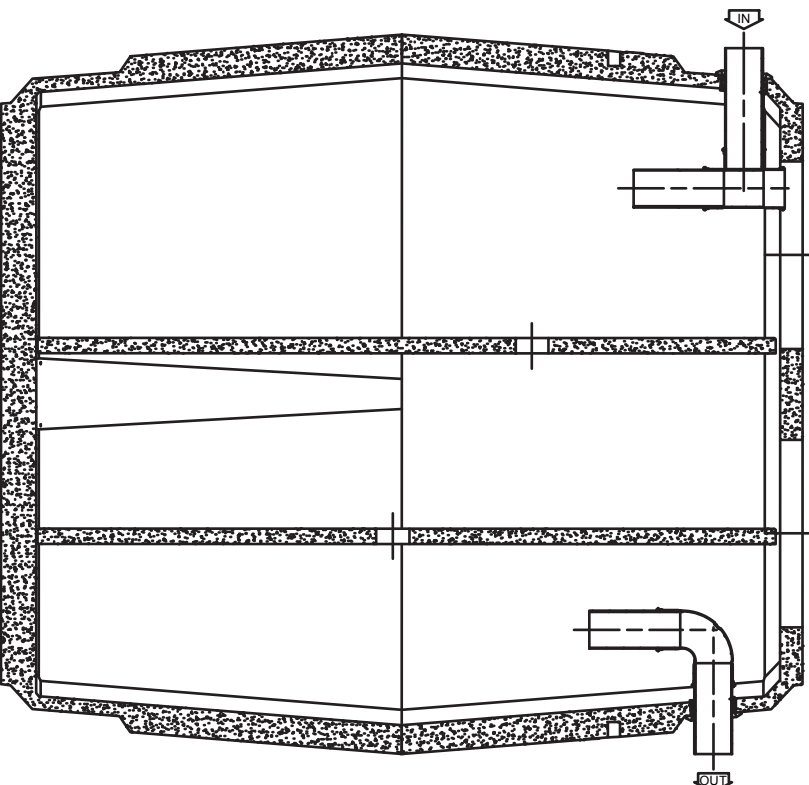
COUPE A-A (1/25)
